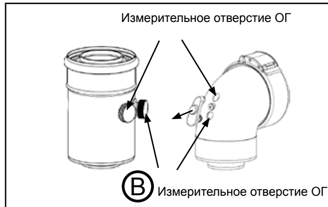
Измерение всасываемого воздуха и параметров ОГ для системы ОГ 60/100 при опциональном исполнении установки
