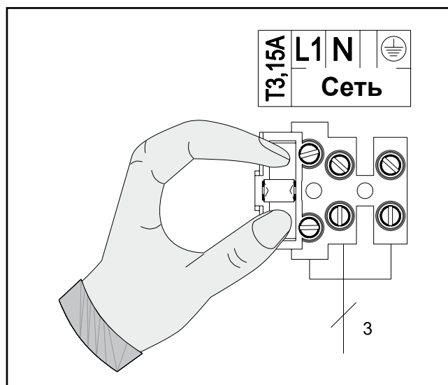
Замена предохранителя
