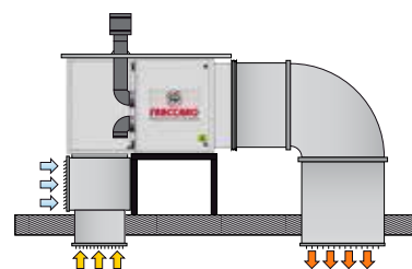
Установка на крыше (требуется комплект для наружного монтажа) Roof top installation (outdoor installation kit required)
