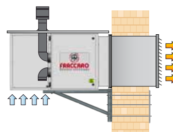
Наружный монтаж в стене Outdoor wall installation
